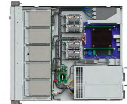
Вид сверху без верхней крышки
